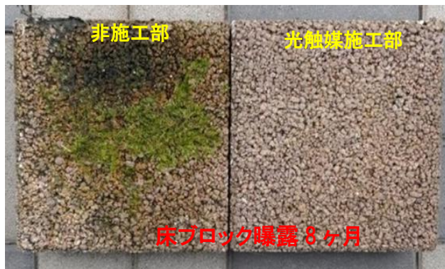
水平での防カビ性能の試験例
