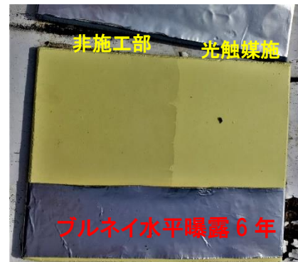
水平セルフクリーニング性能の試験
